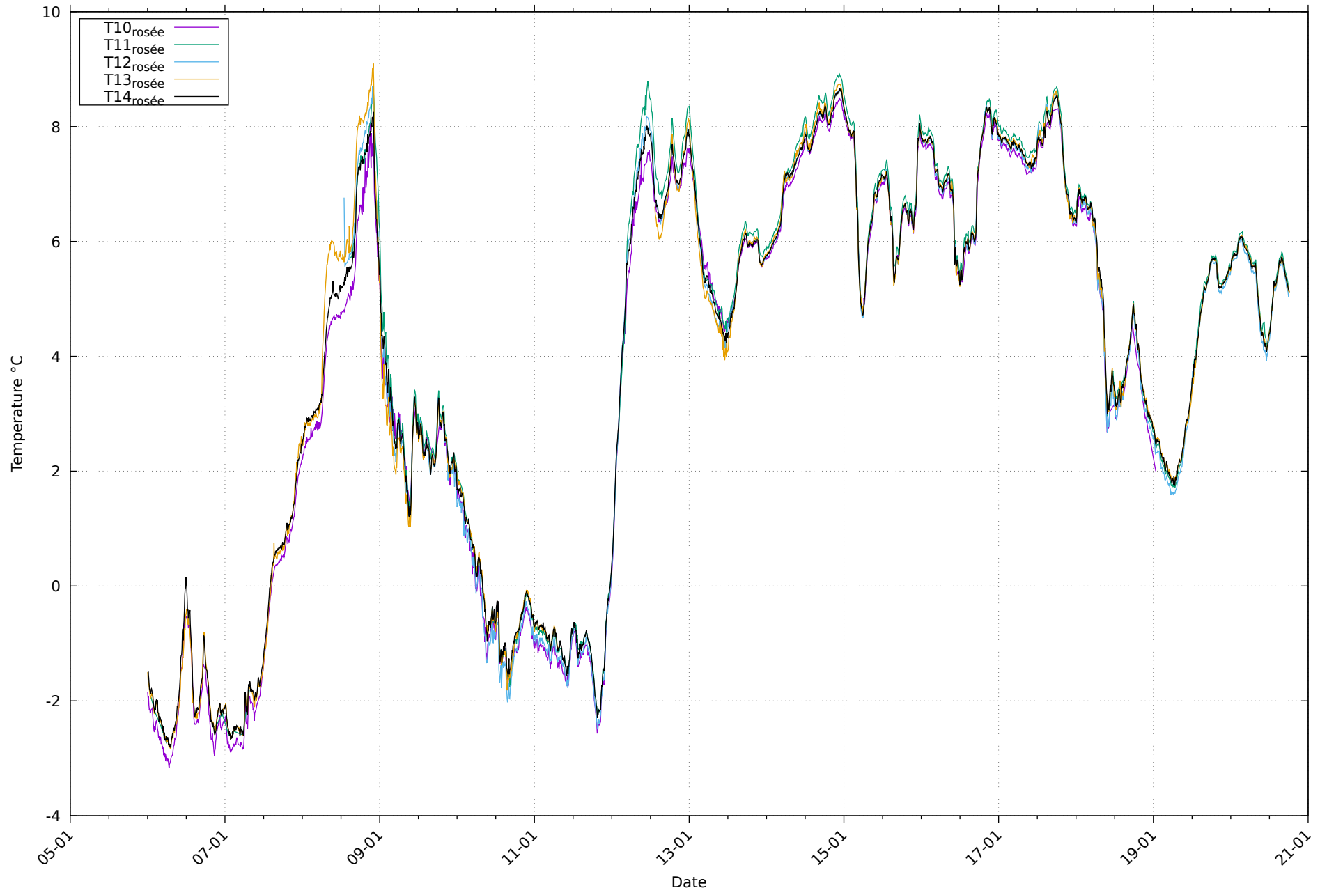
Températures de rosée au 25/01/2026
