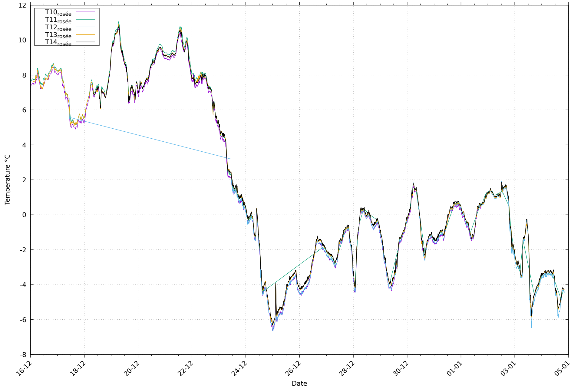
Températures de rosée au 04/01/2026
