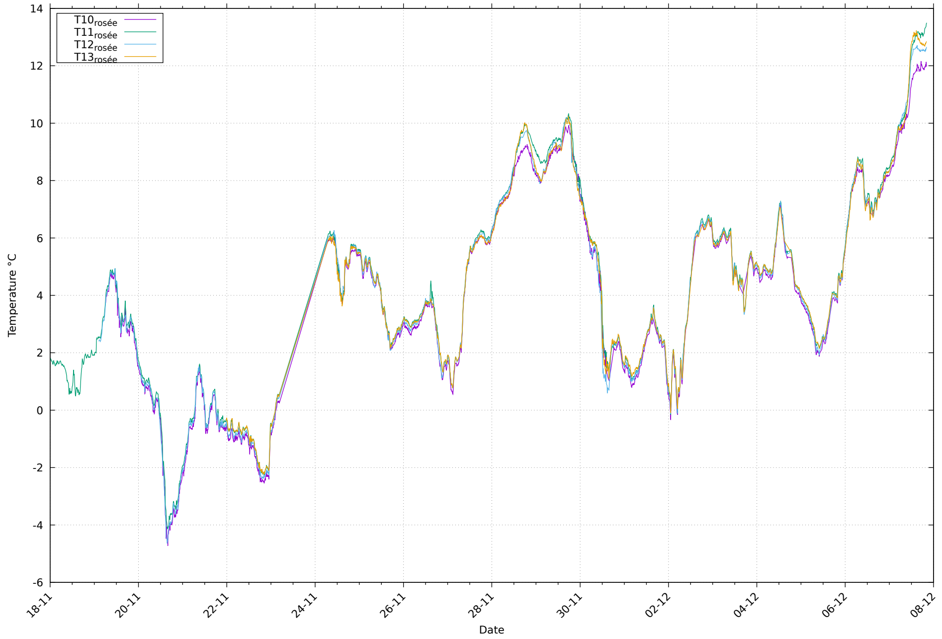
Températures de rosée au 07/12/2025
