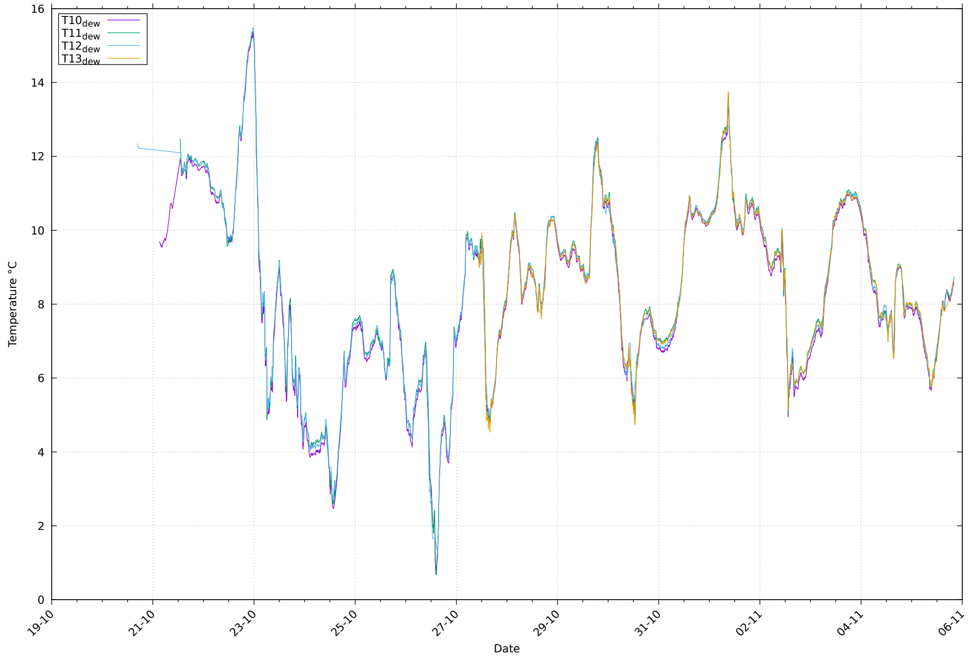
Températures de rosée au 09/11/2025
