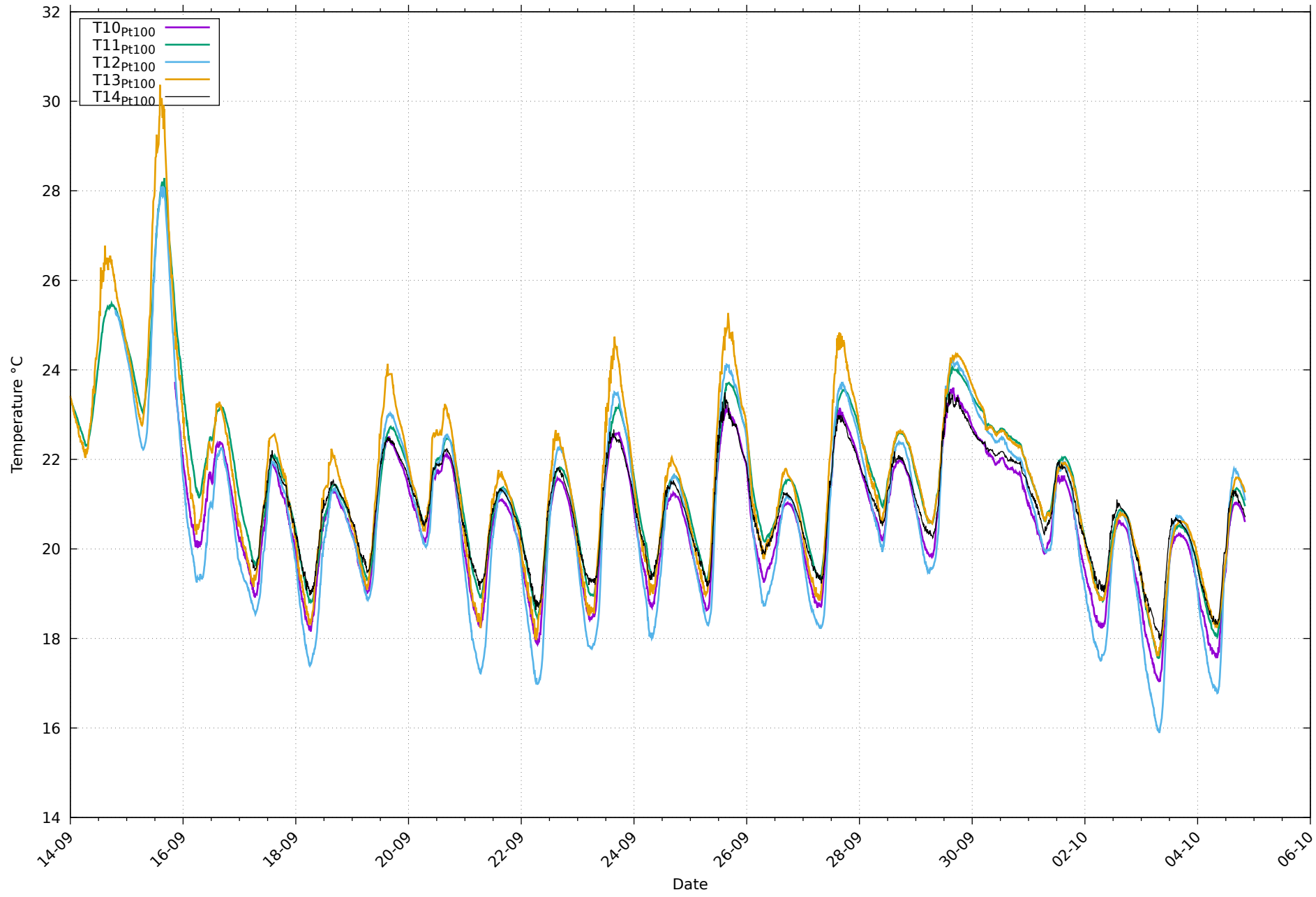
Températures de paroi Pt100 au 04/10/2026
