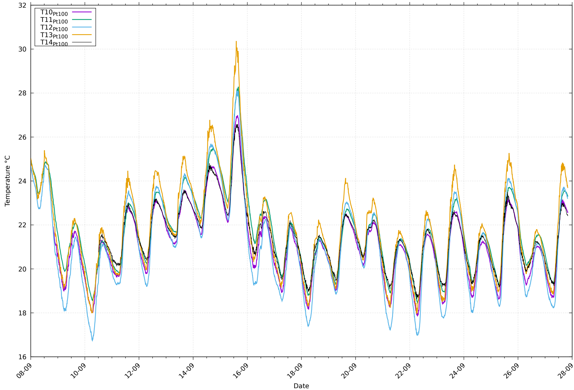
Températures de paroi Pt100 au 27/09/2026
