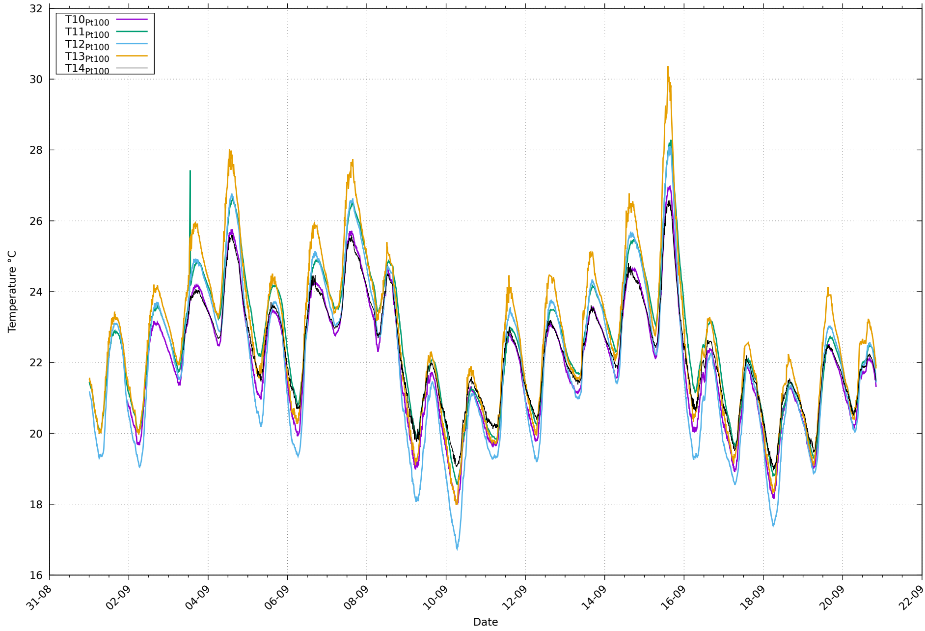
Températures de paroi Pt100 au 20/09/2026
