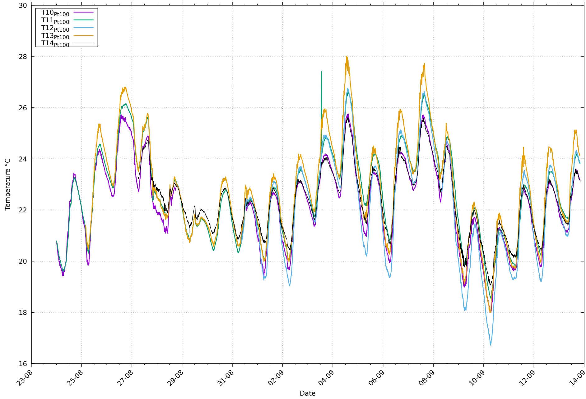
Températures de paroi Pt100 au 13/09/2026
