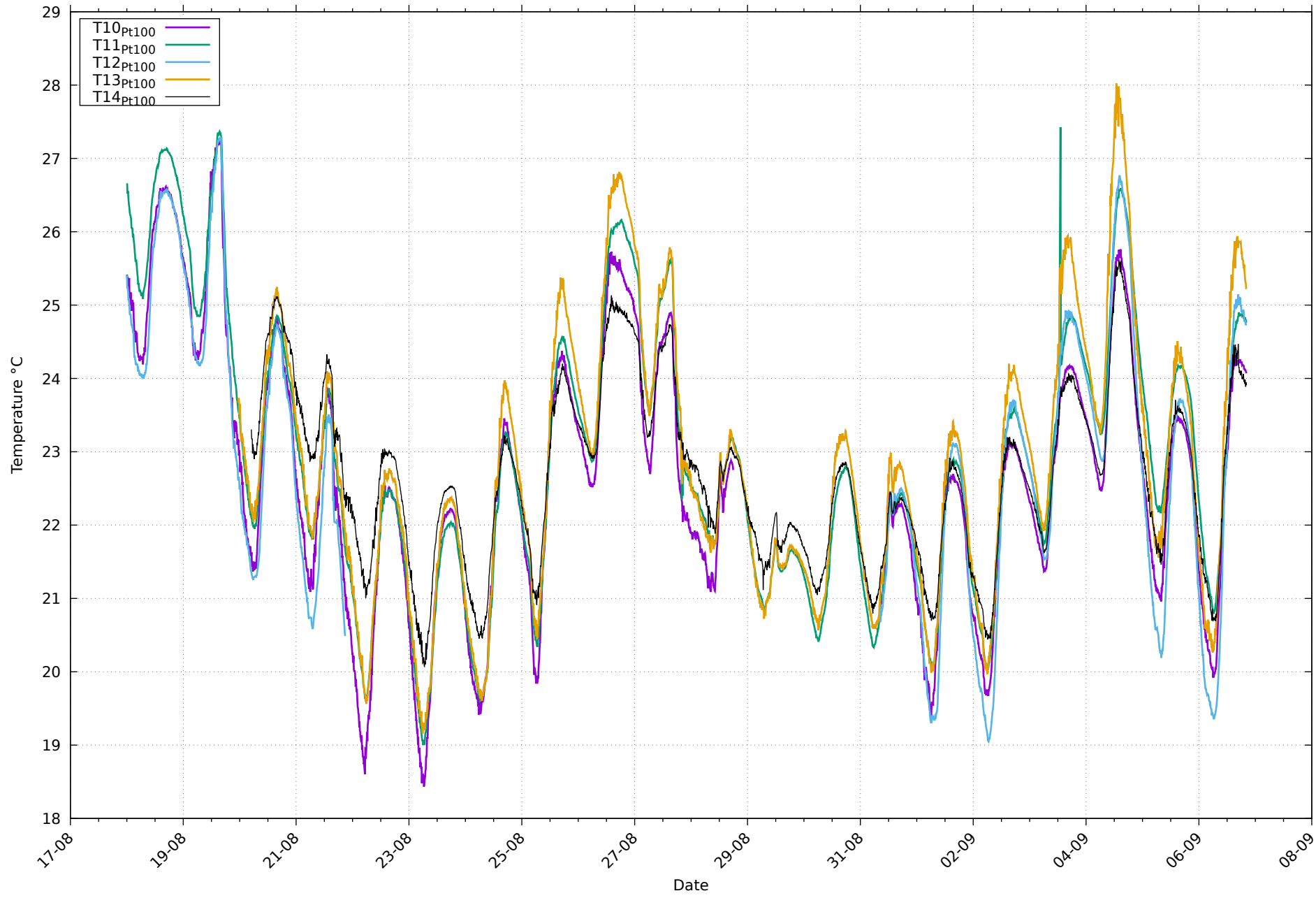
Températures de paroi Pt100 au 06/09/2026
