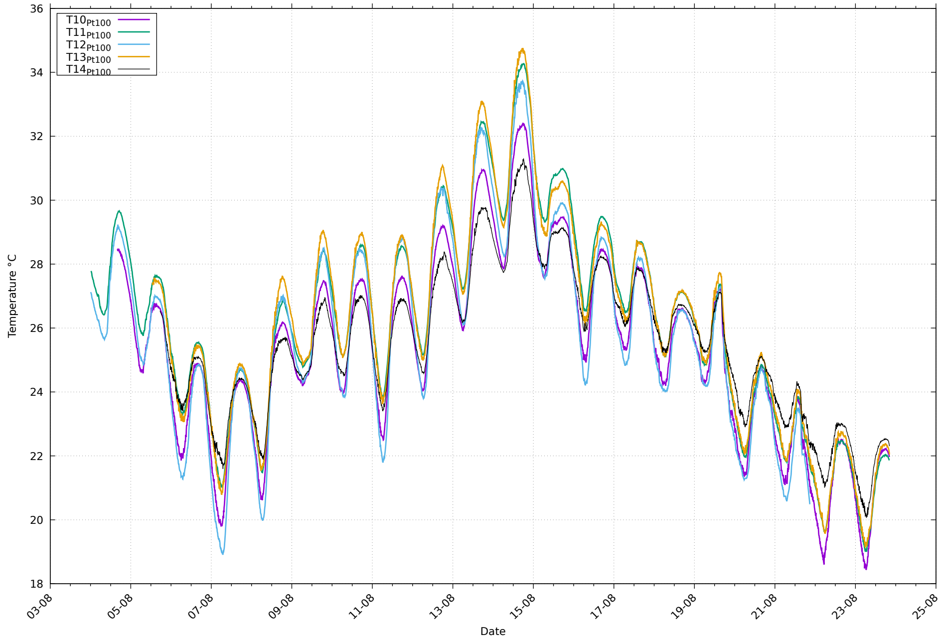
Températures de paroi Pt100 au 23/08/2026
