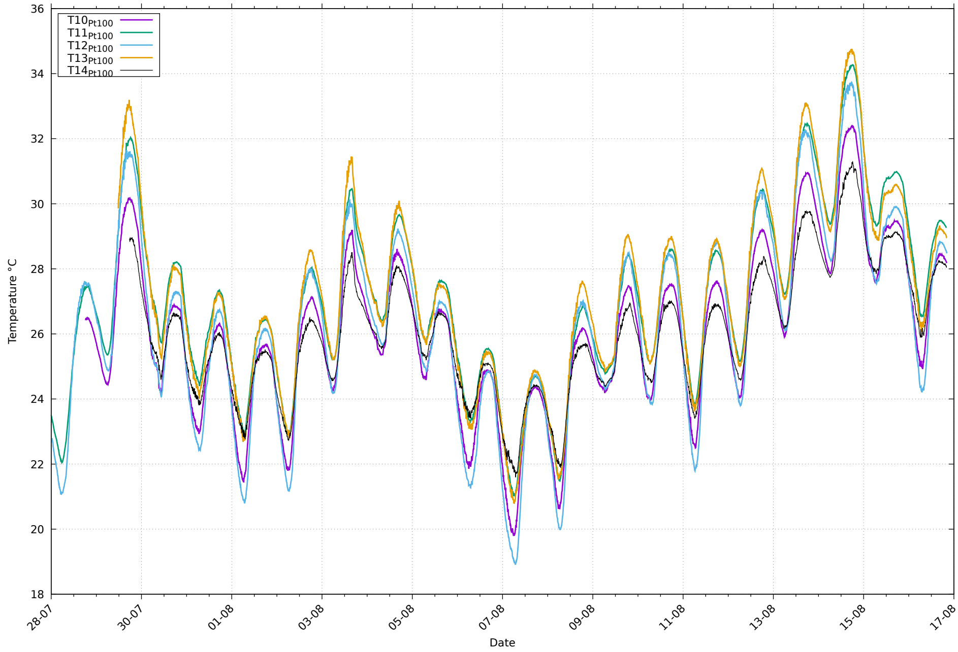
Températures de paroi Pt100 au 16/08/2026
