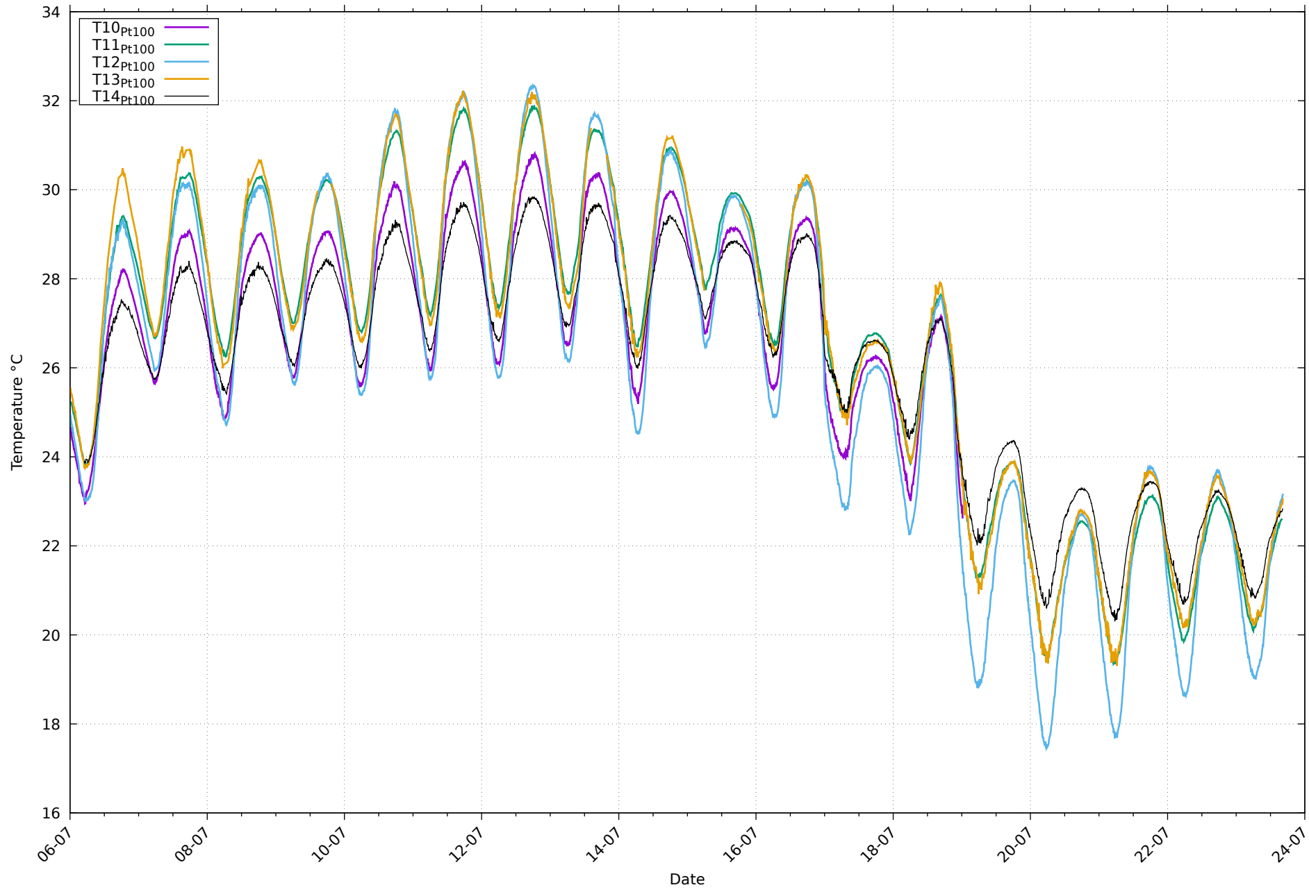
Températures de paroi Pt100 au 26/07/2026
