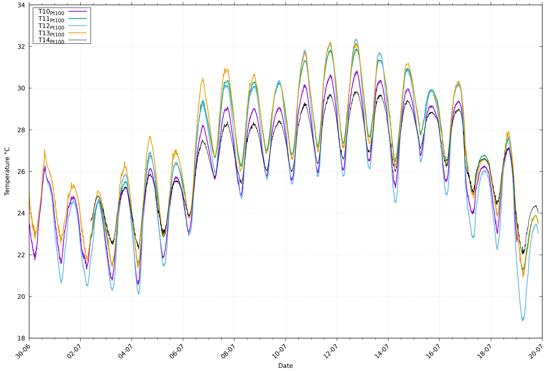
Températures de paroi Pt100 au 19/07/2026
