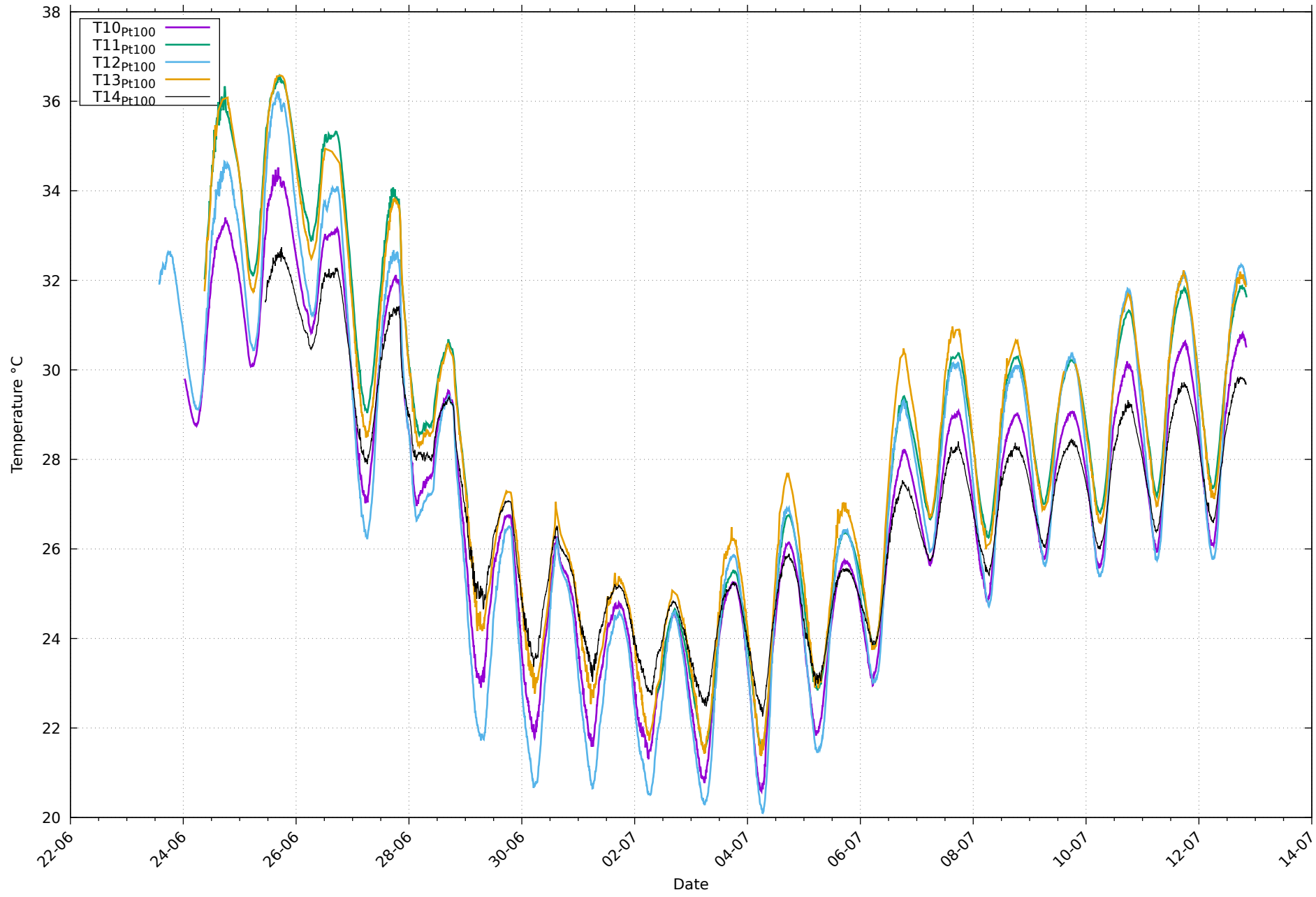
Températures de paroi Pt100 au 12/07/2026
