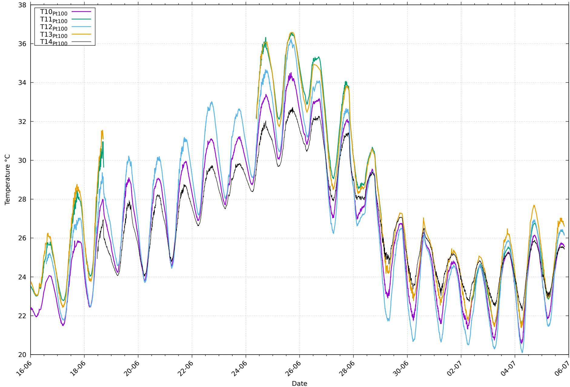
Températures de paroi Pt100 au 05/07/2026
