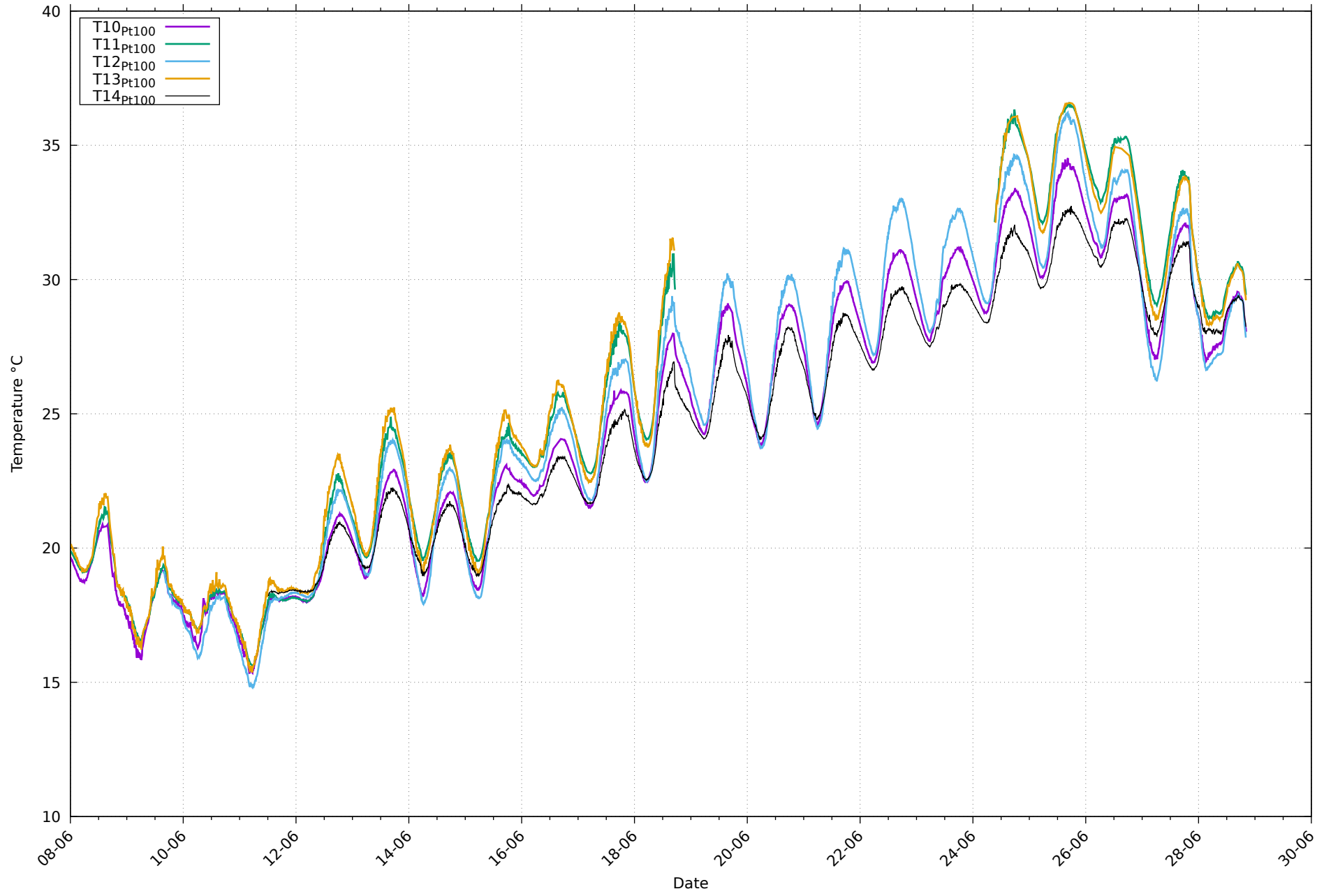
Températures de paroi Pt100 au 28/06/2026
