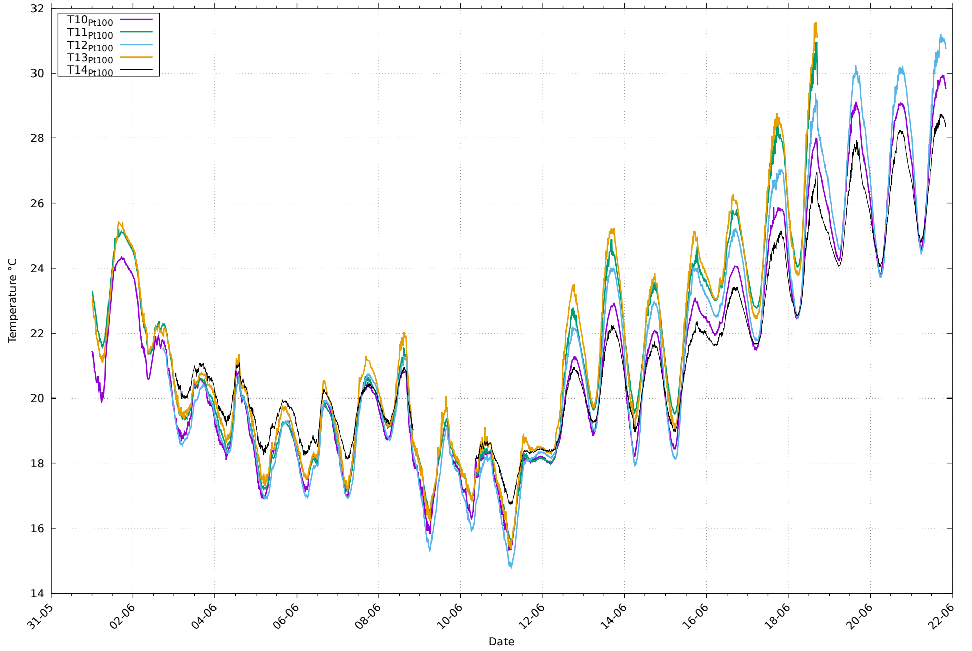
Températures de paroi Pt100 au 21/06/2026
