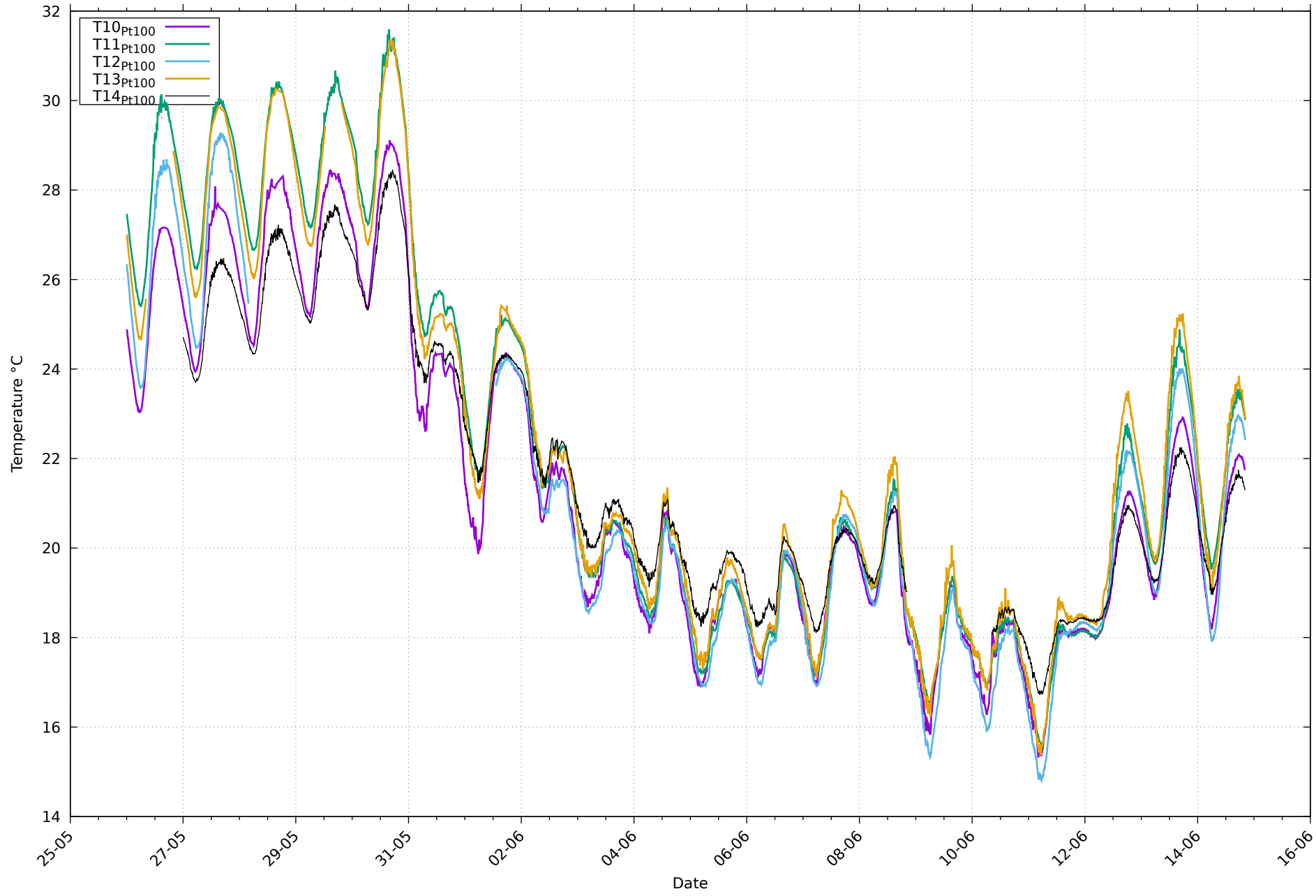
Températures de paroi Pt100 au 14/06/2026
