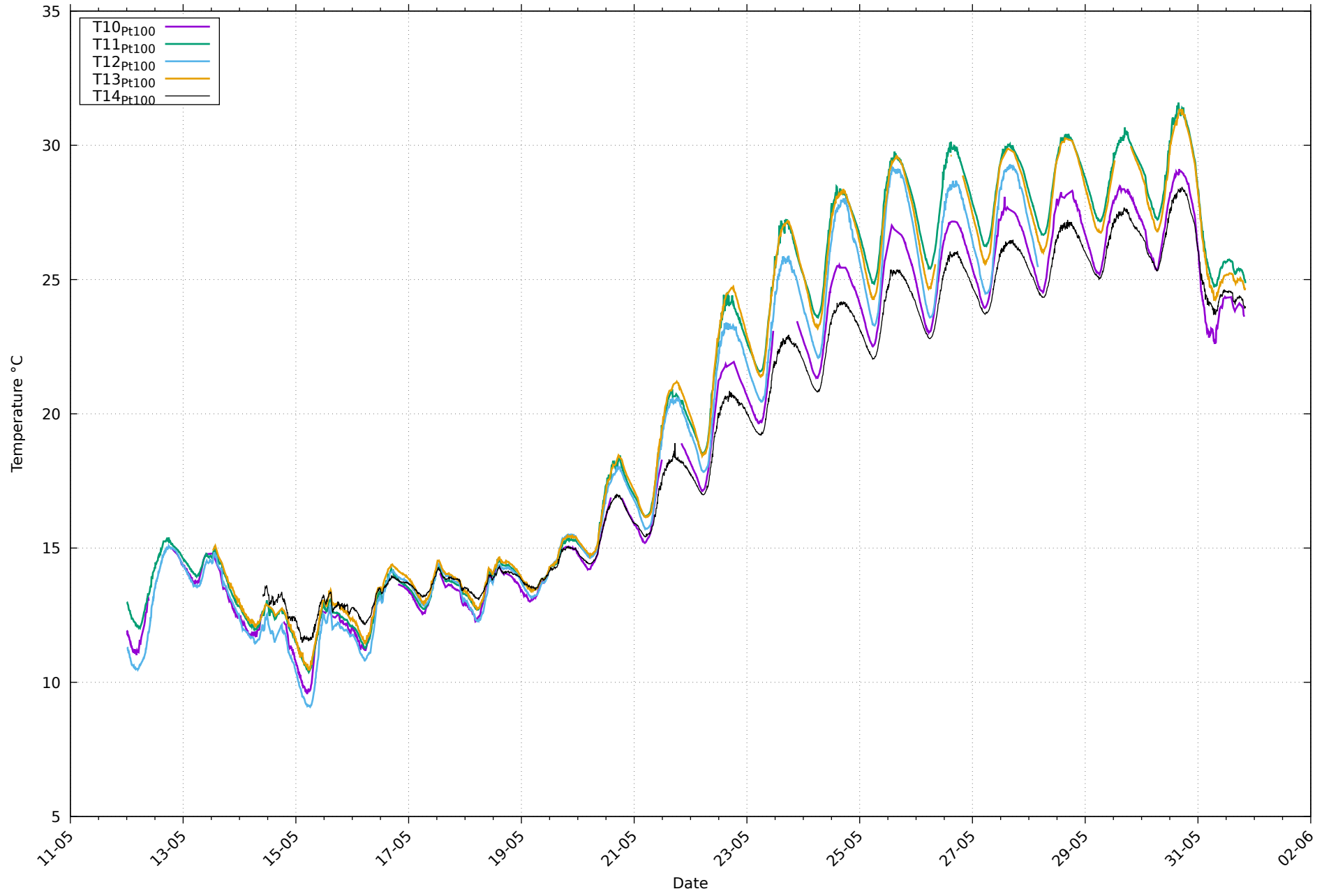
Températures de paroi Pt100 au 31/05/2026
