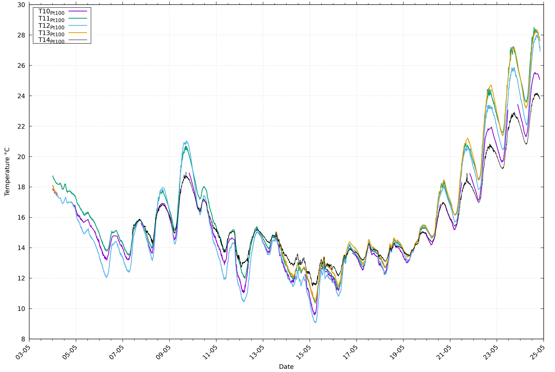
Températures de paroi Pt100 au 24/05/2026
