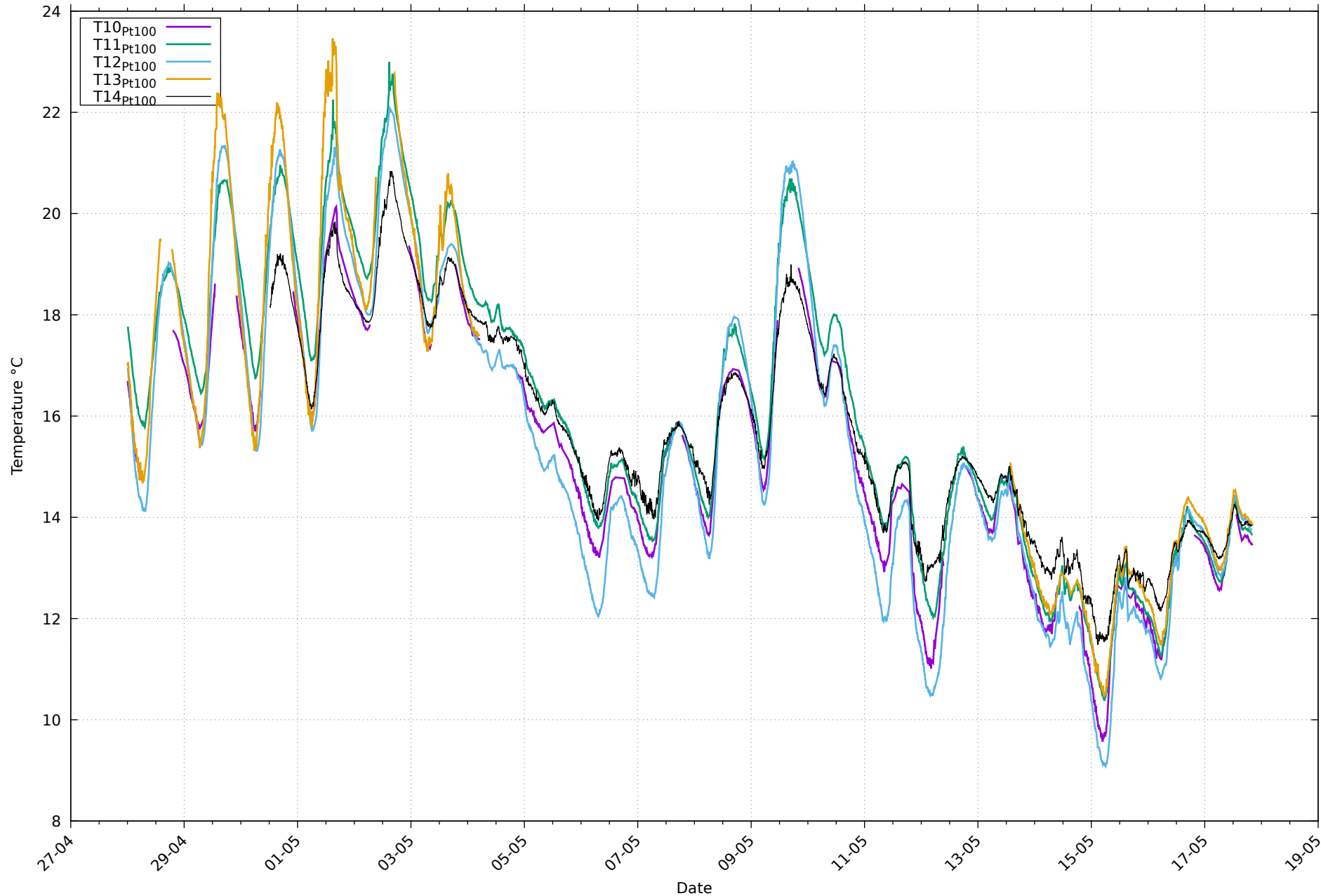
Températures de paroi Pt100 au 17/05/2026
