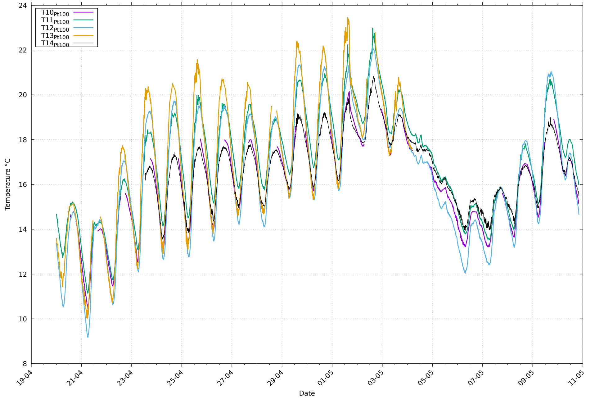
Températures de paroi Pt100 au 10/05/2026
