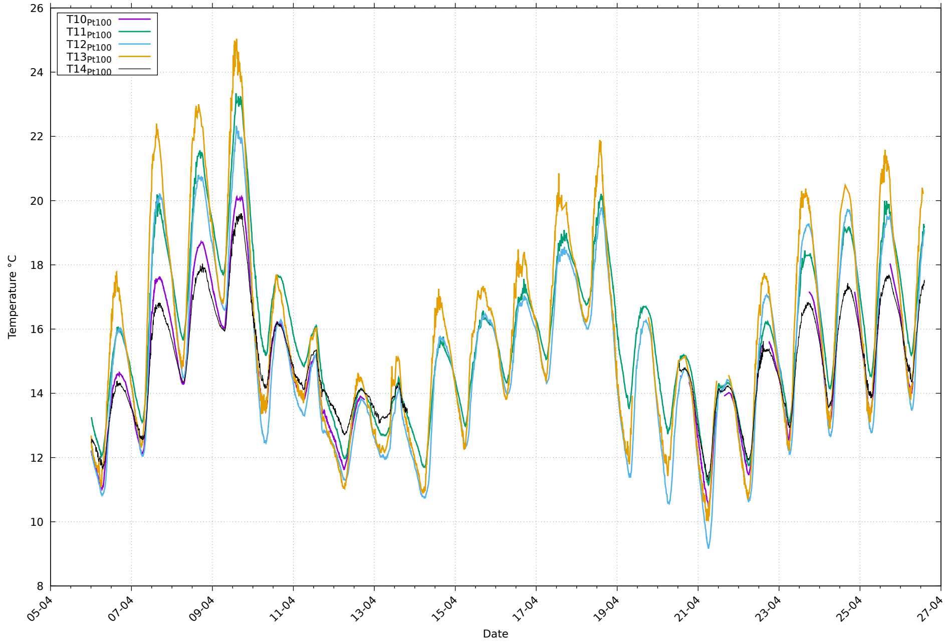
Températures de paroi Pt100 au 26/04/2026
