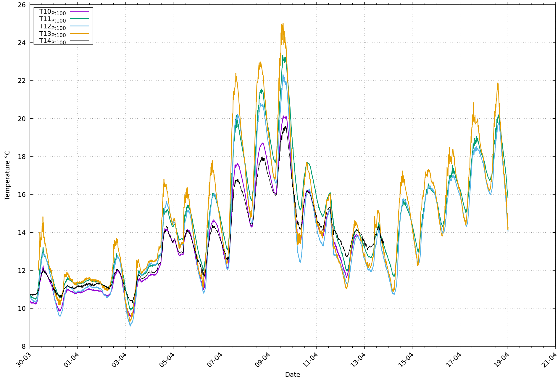
Températures de paroi Pt100 au 19/04/2026
