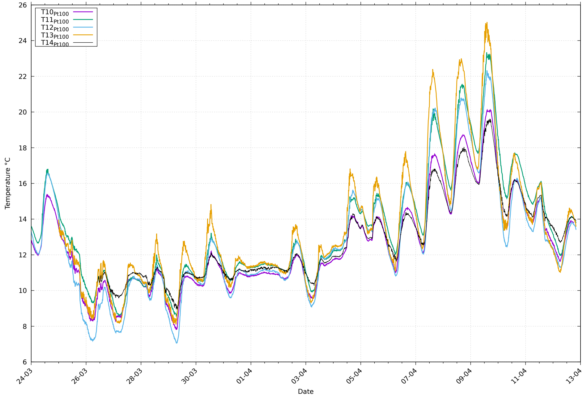
Températures de paroi Pt100 au 12/04/2026
