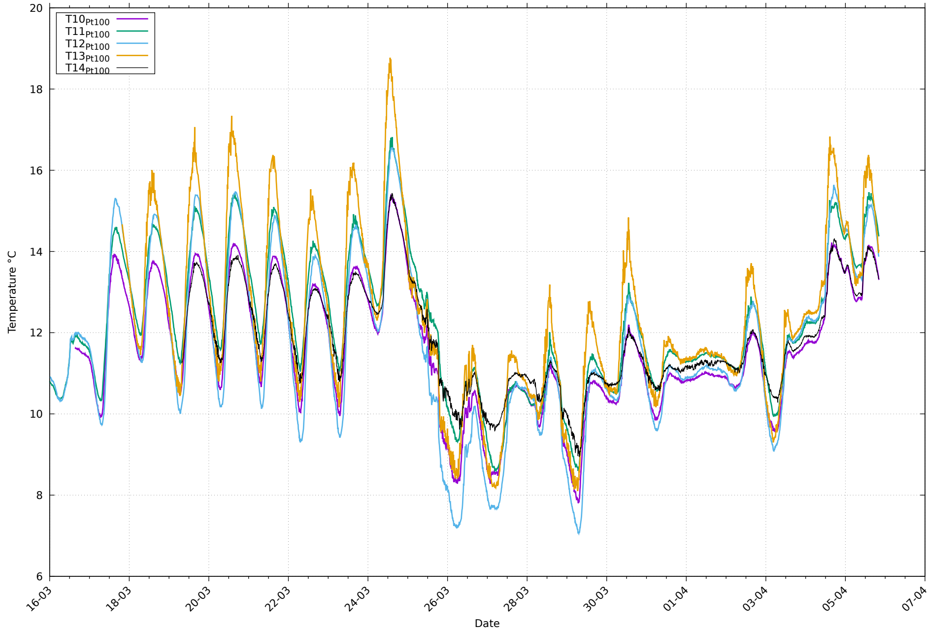
Températures de paroi Pt100 au 05/04/2026
