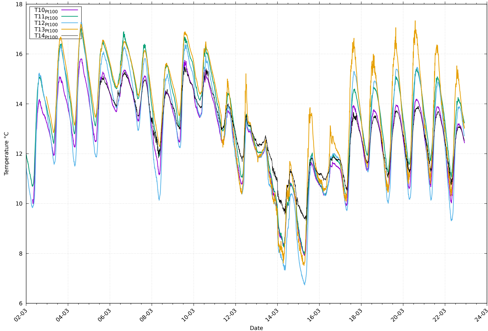
Températures de paroi Pt100 au 22/03/2026
