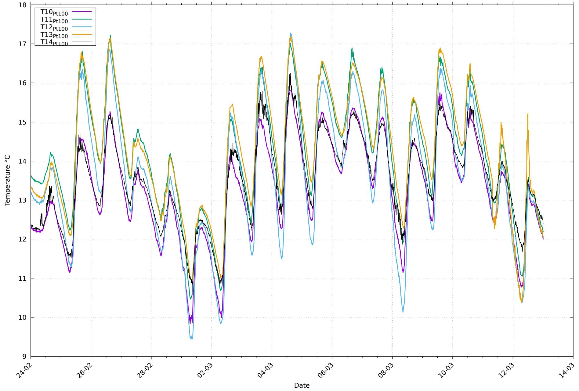
Températures de paroi Pt100 au 15/03/2026
