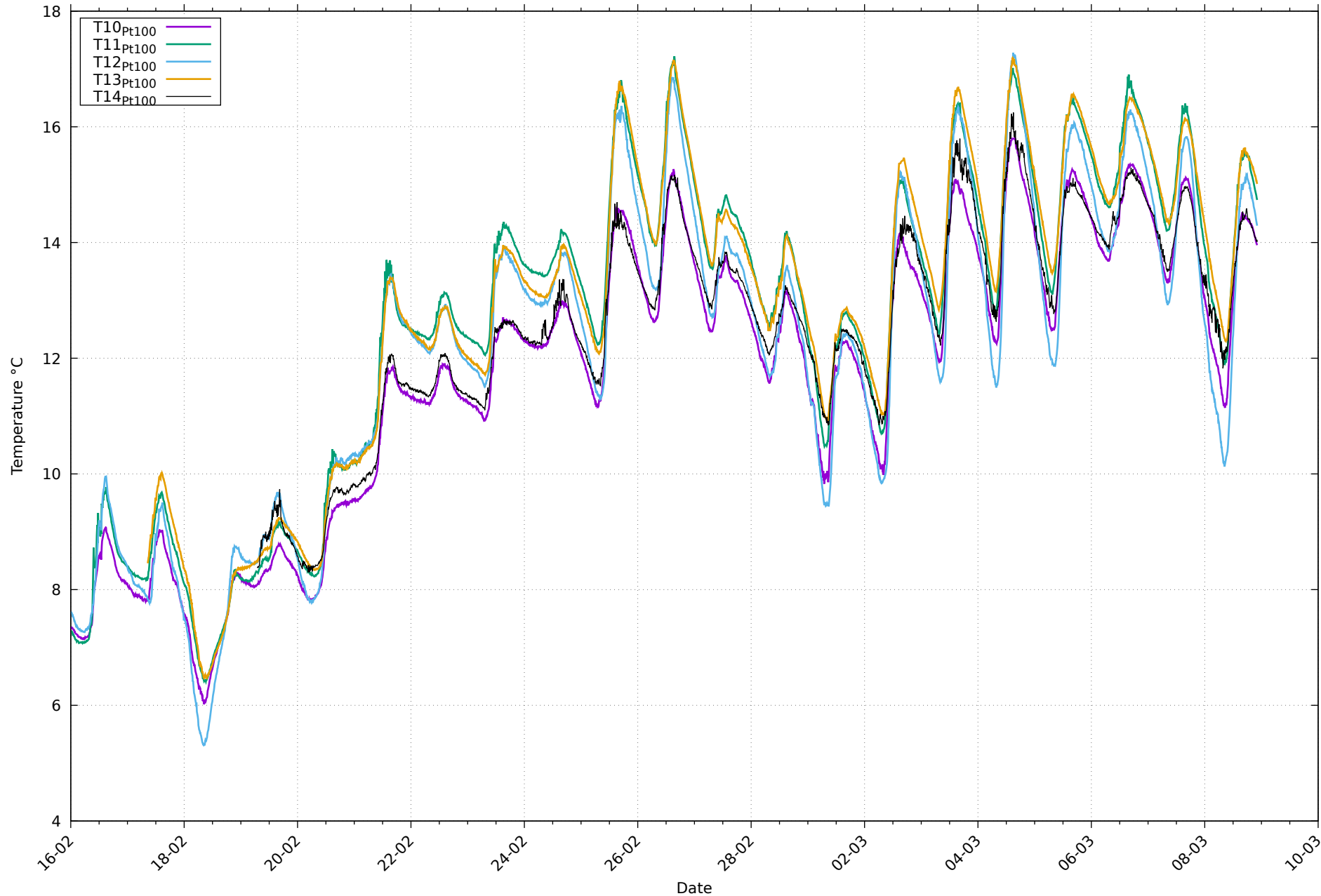
Températures de paroi Pt100 au 08/03/2026
