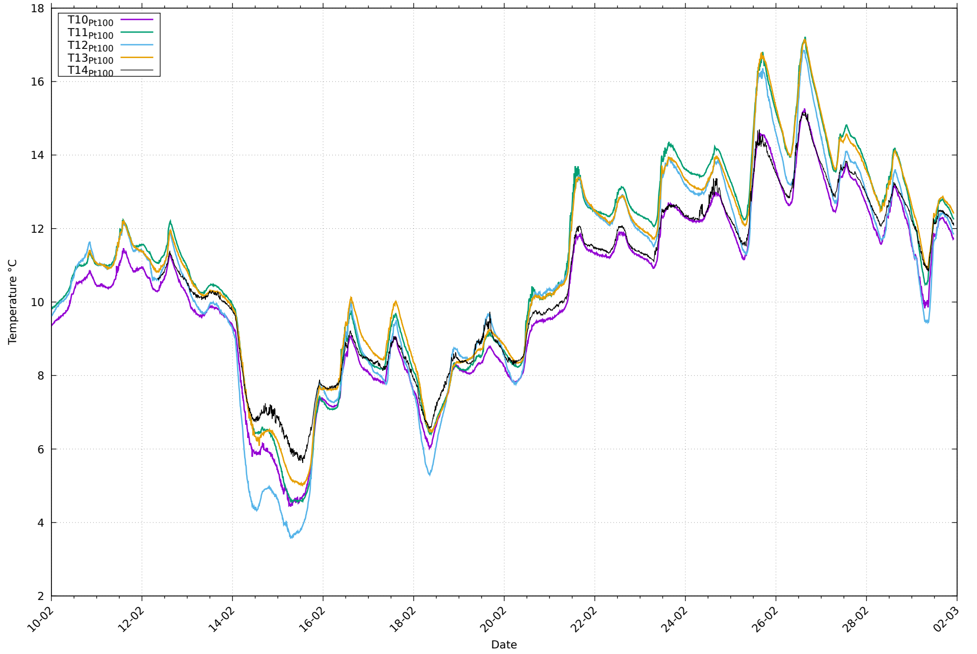
Températures de paroi Pt100 au 01/03/2026
