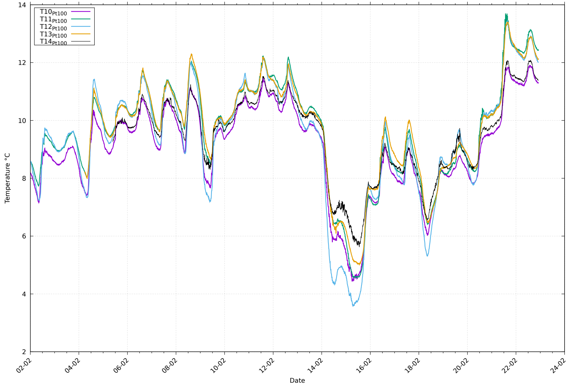
Températures de paroi Pt100 au 22/02/2026
