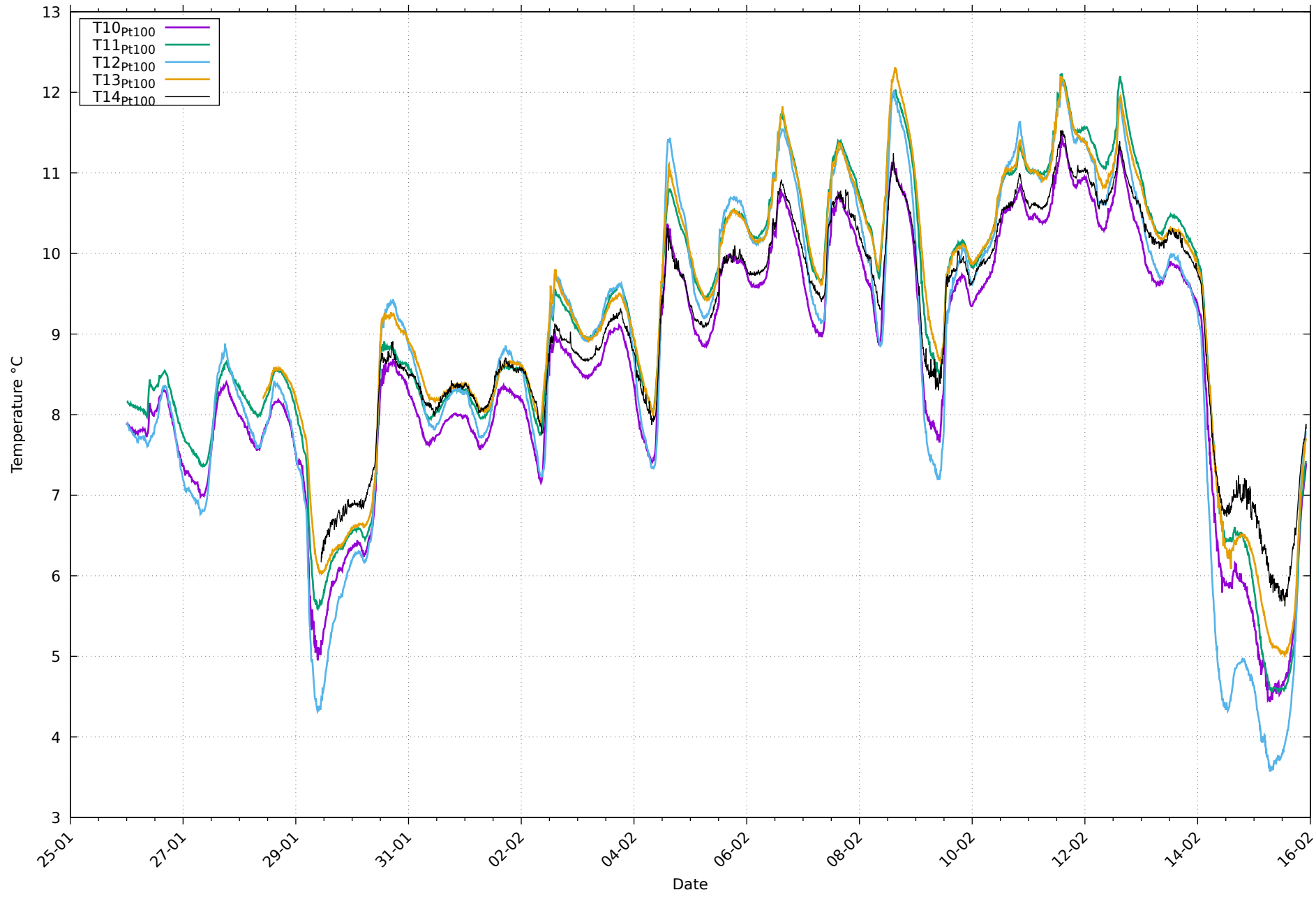
Températures de paroi Pt100 au 15/02/2026
