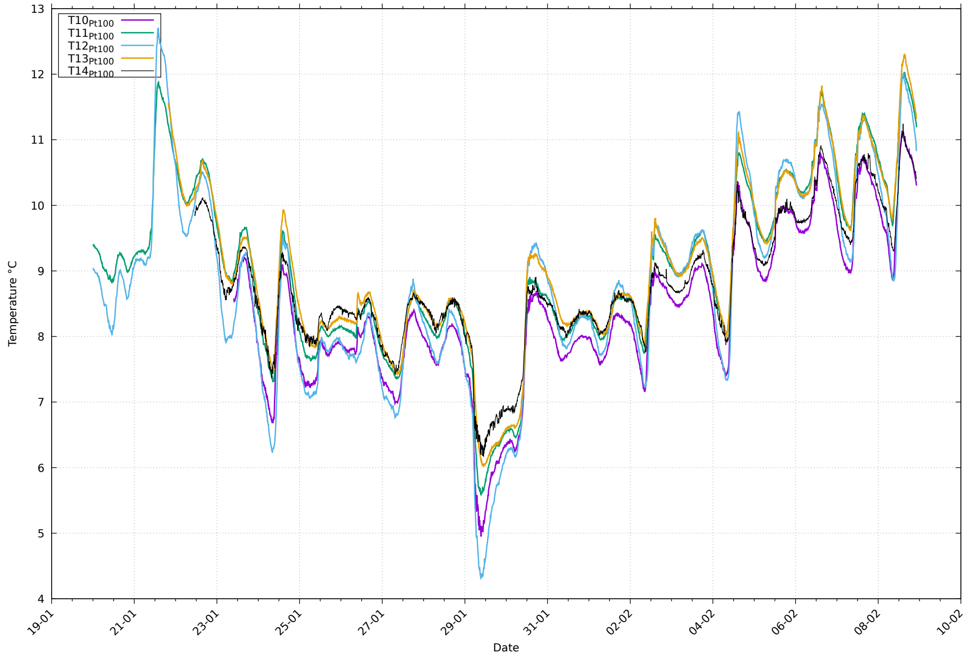
Températures de paroi Pt100 au 08/02/2026
