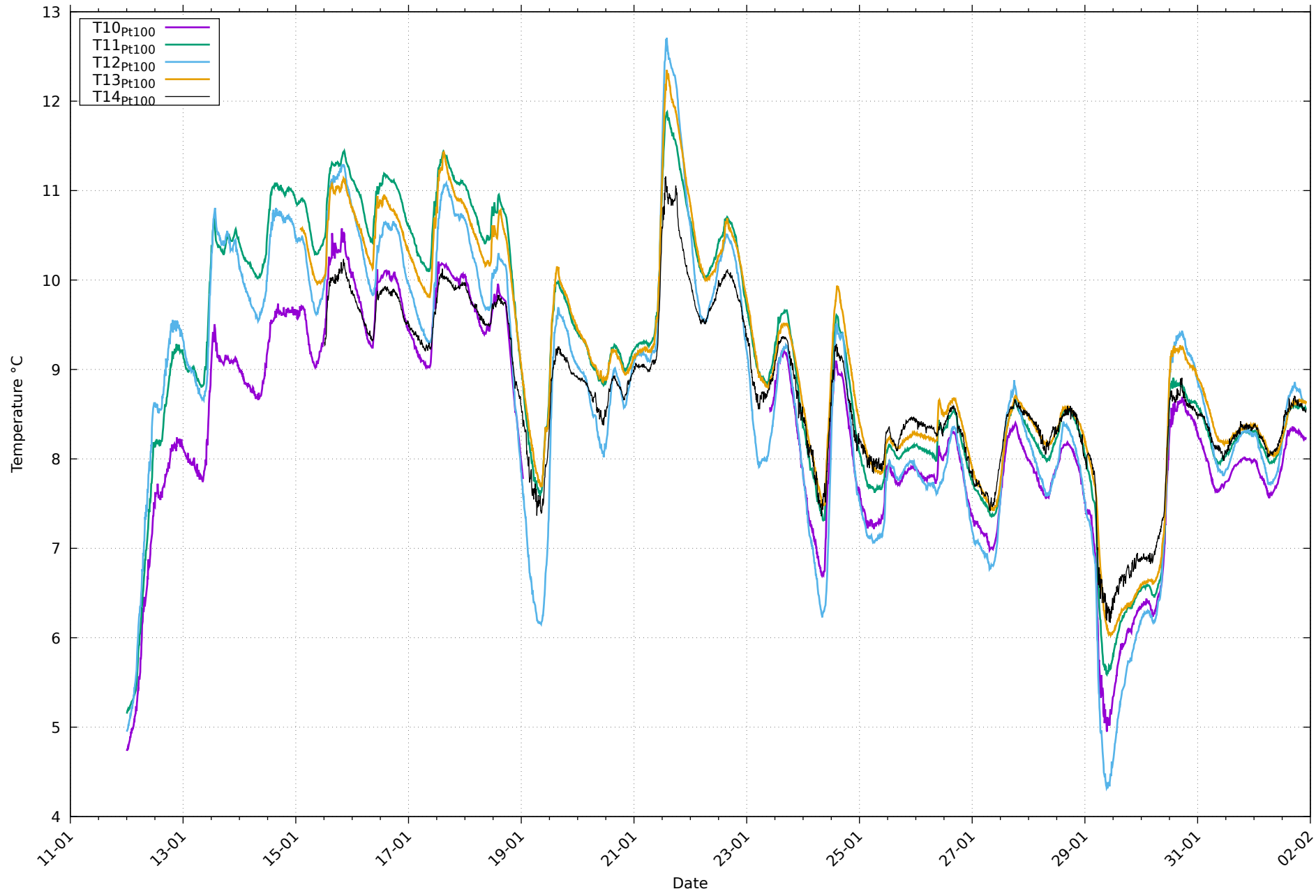
Températures de paroi Pt100 au 01/02/2026
