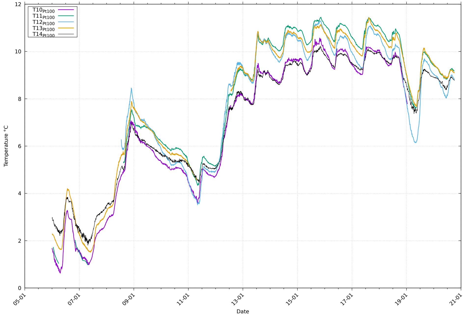
Températures de paroi Pt100 au 25/01/2026
