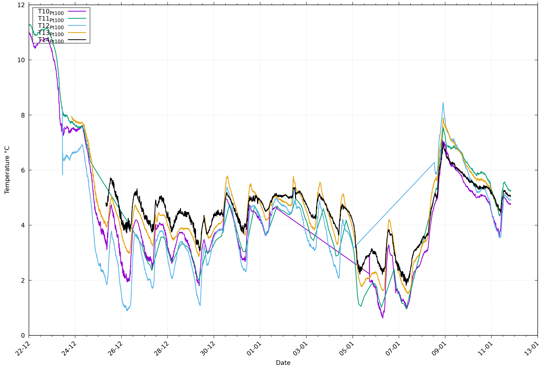
Températures de paroi Pt100 au 11/01/2026
