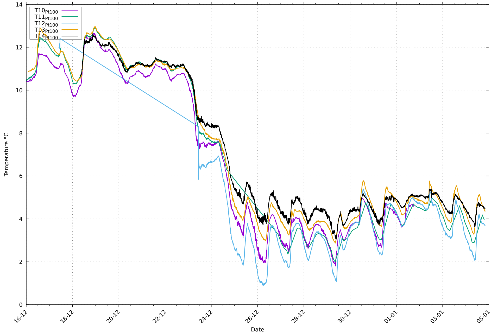
Températures de paroi Pt100 au 04/01/2026
