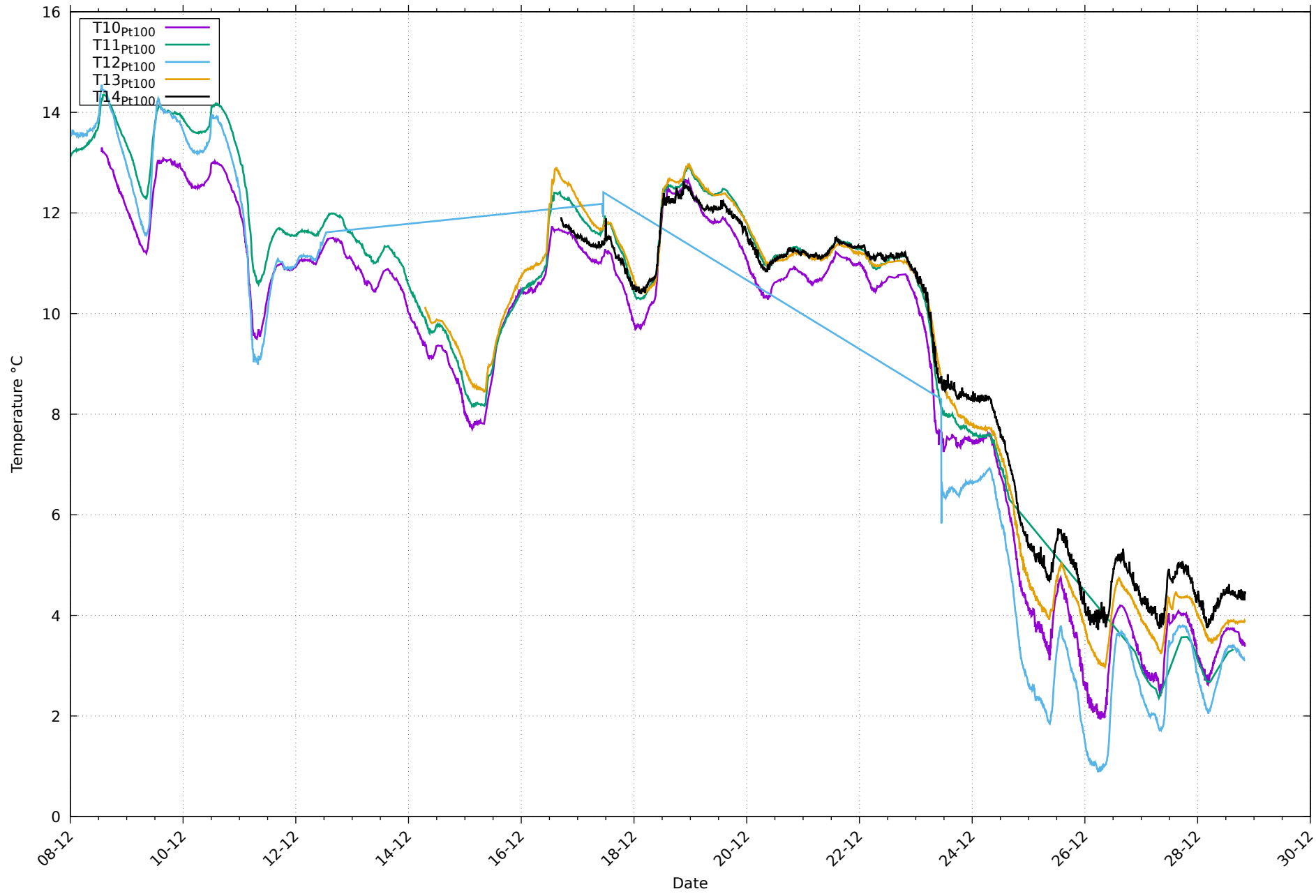
Températures de paroi Pt100 au 28/12/2025
