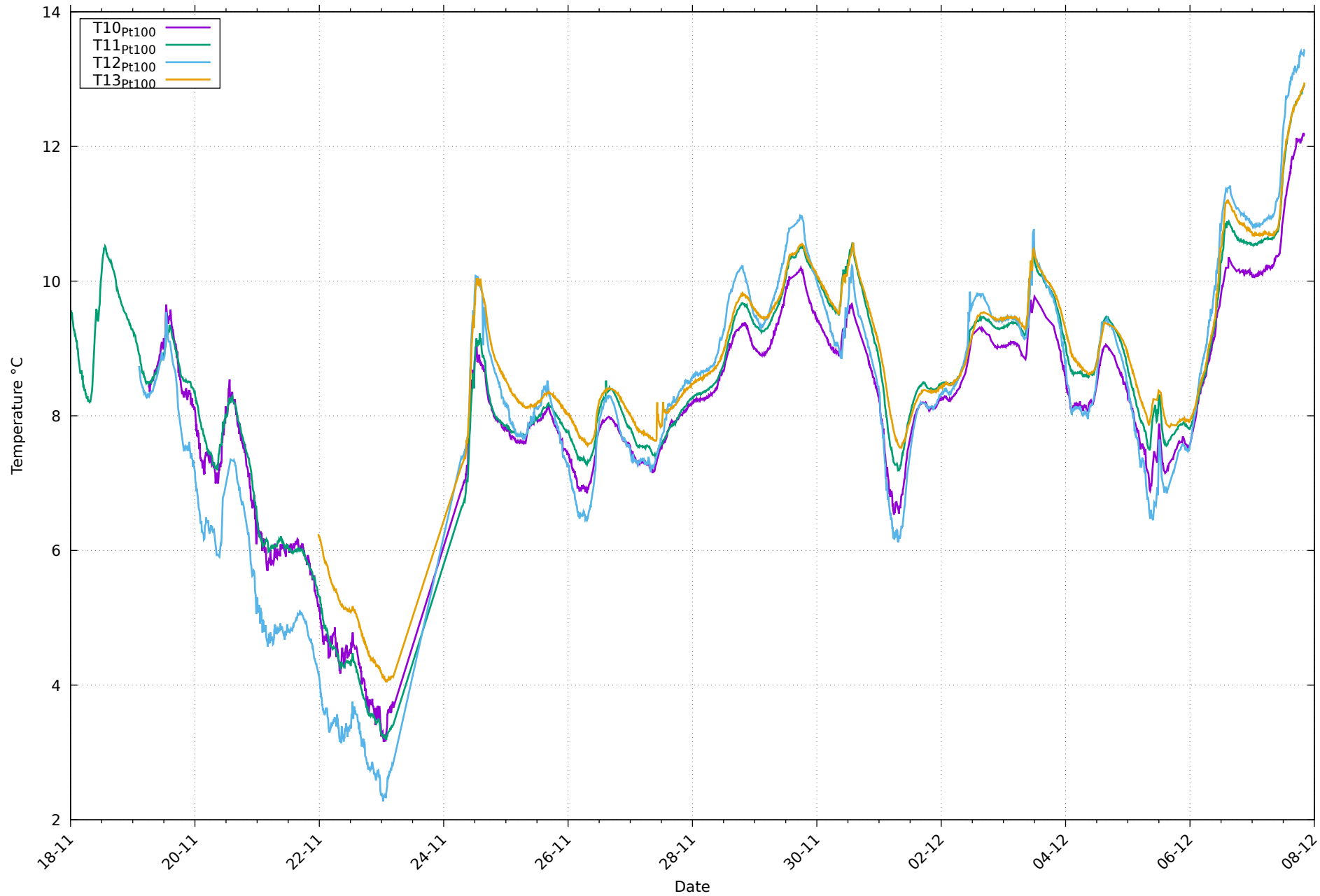
Températures de paroi Pt100 au 07/12/2025
