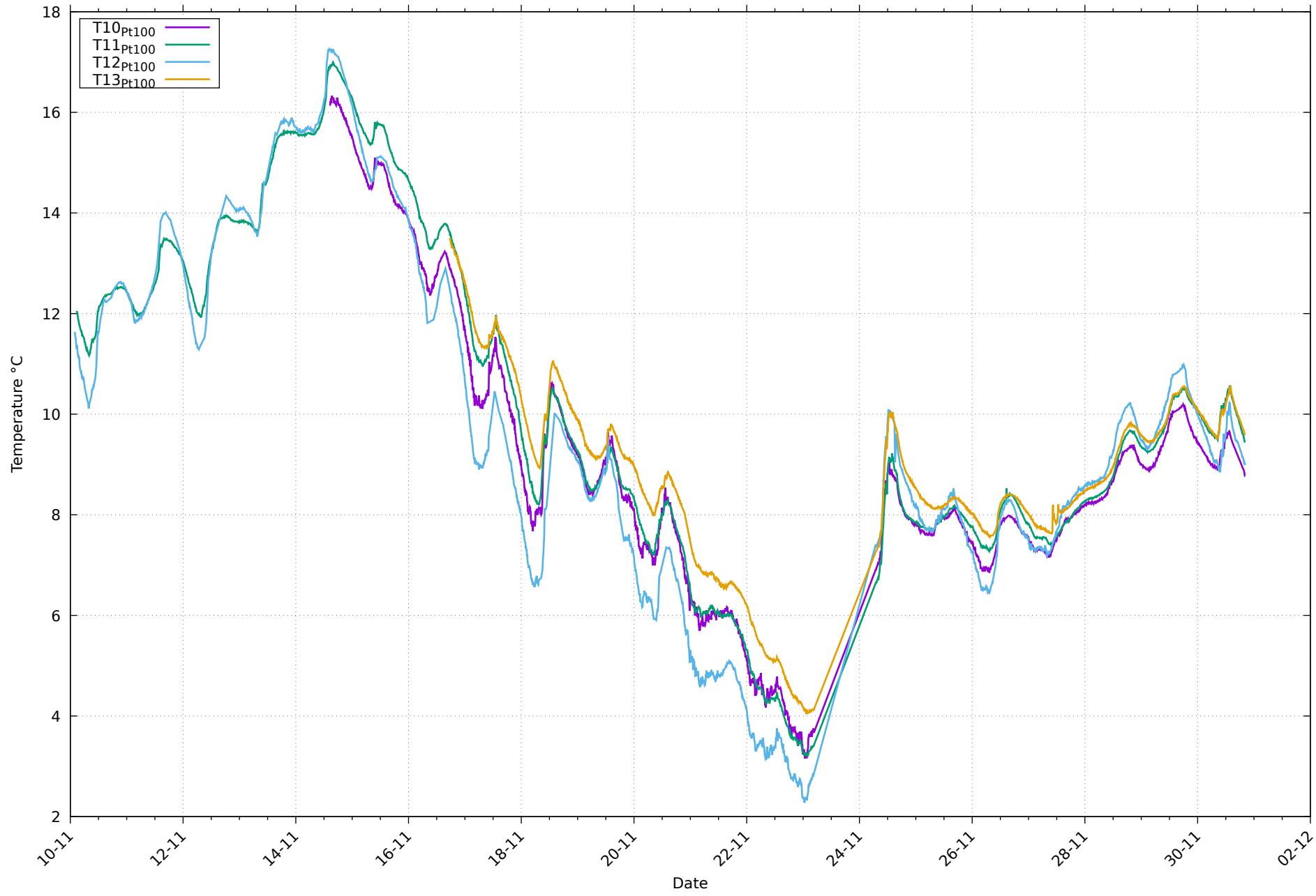
Températures de paroi Pt100 au 30/11/2025
