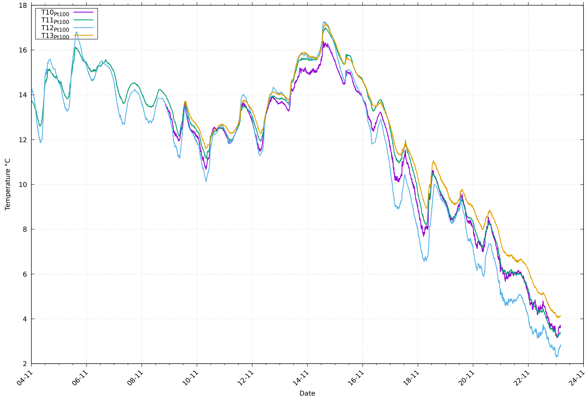
Températures de paroi Pt100 au 23/11/2025
