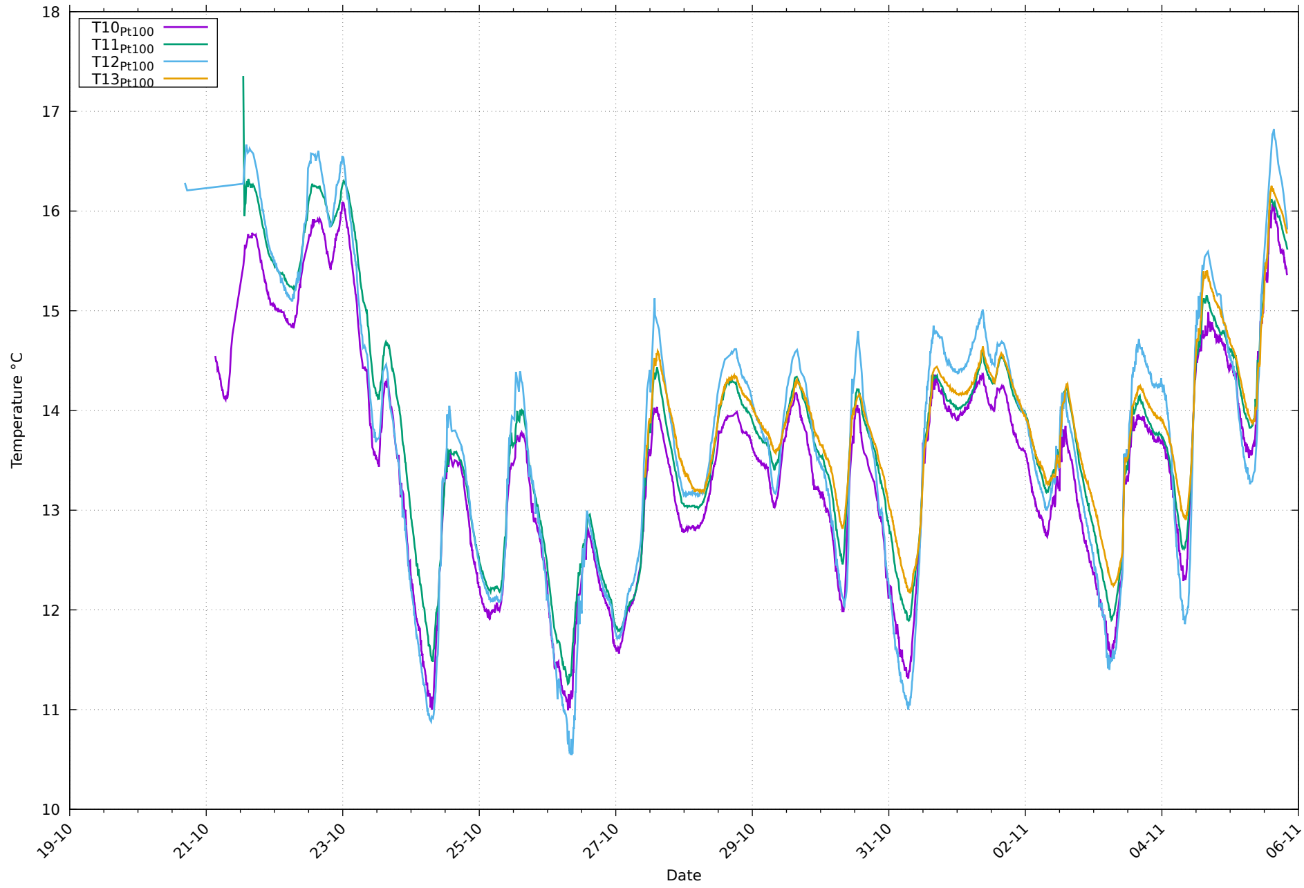
Températures de paroi Pt100 au 09/11/2025
