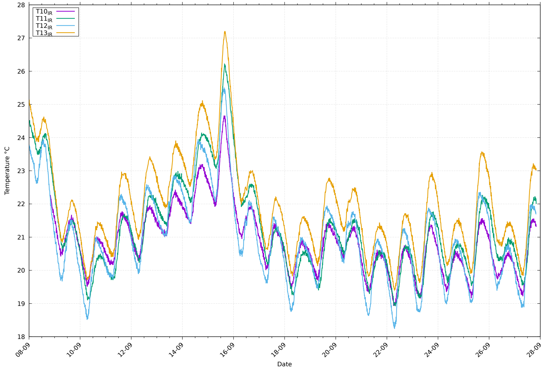
Températures de paroi IR au 27/09/2026
