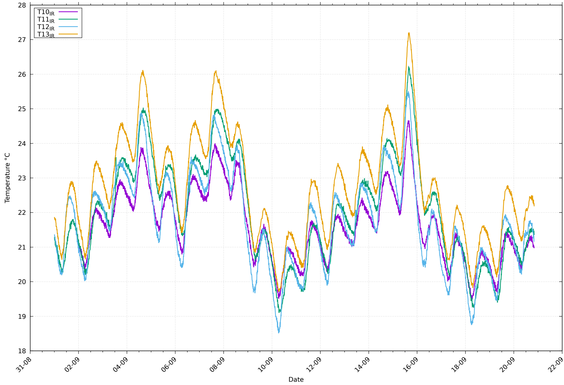
Températures de paroi IR au 20/09/2026
