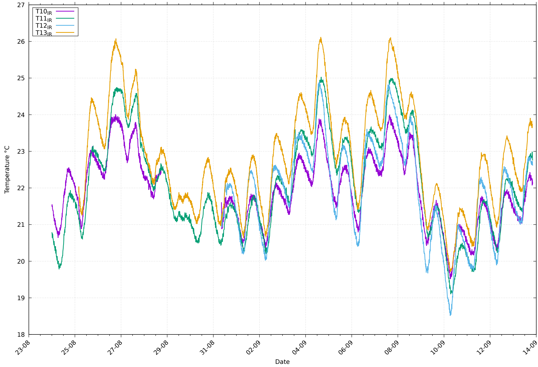
Températures de paroi IR au 13/09/2026
