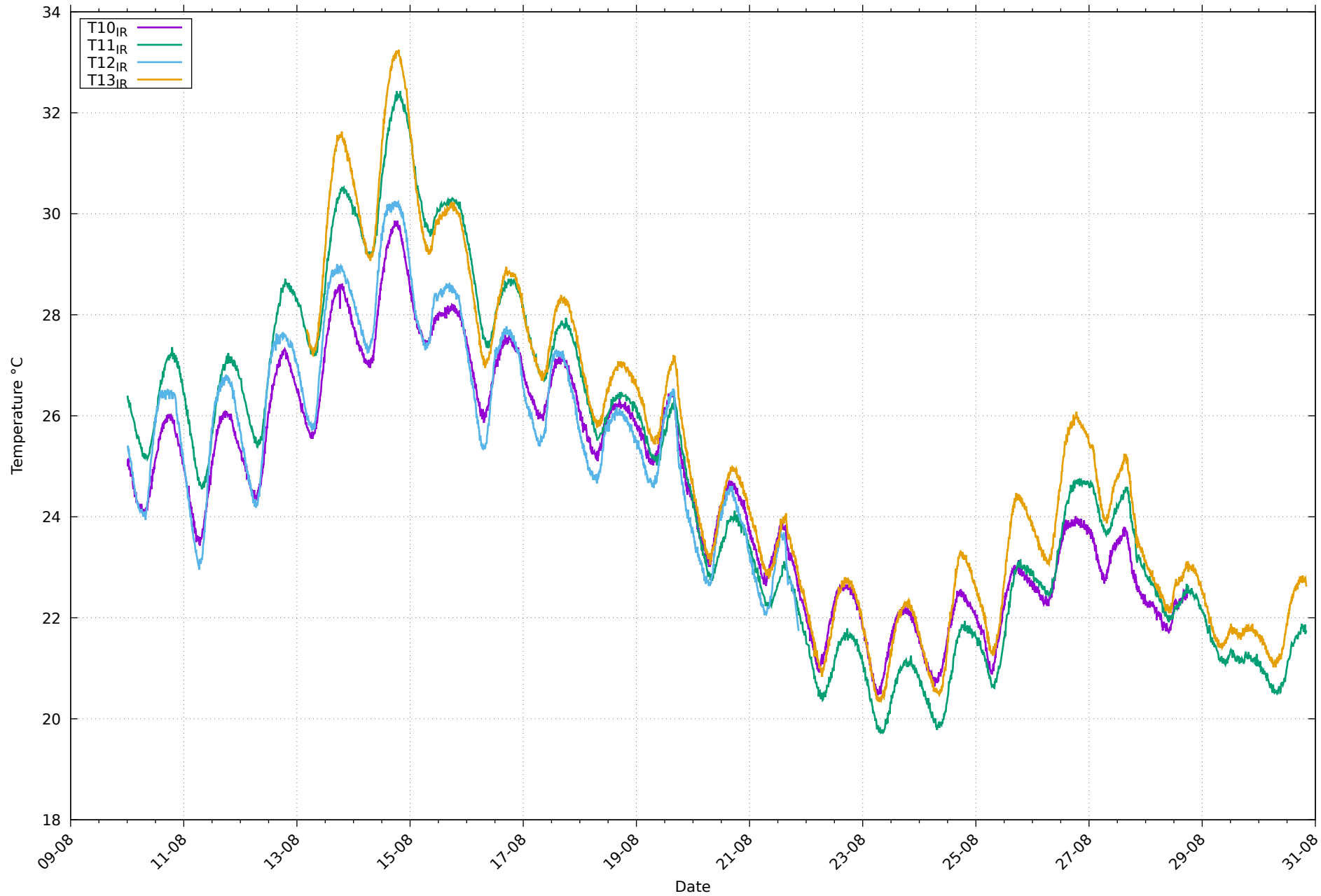
Températures de paroi IR au 30/08/2026
