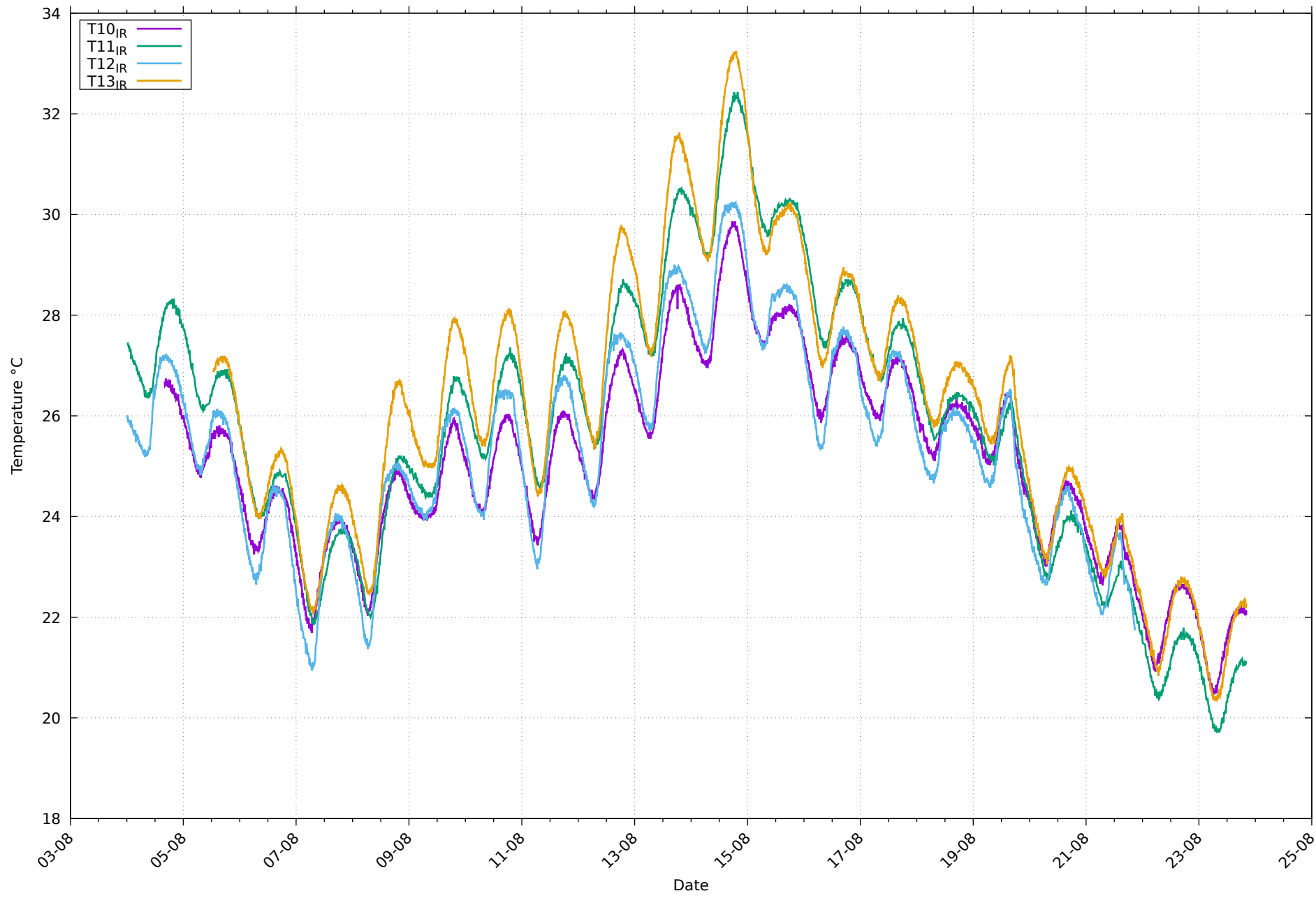
Températures de paroi IR au 23/08/2026
