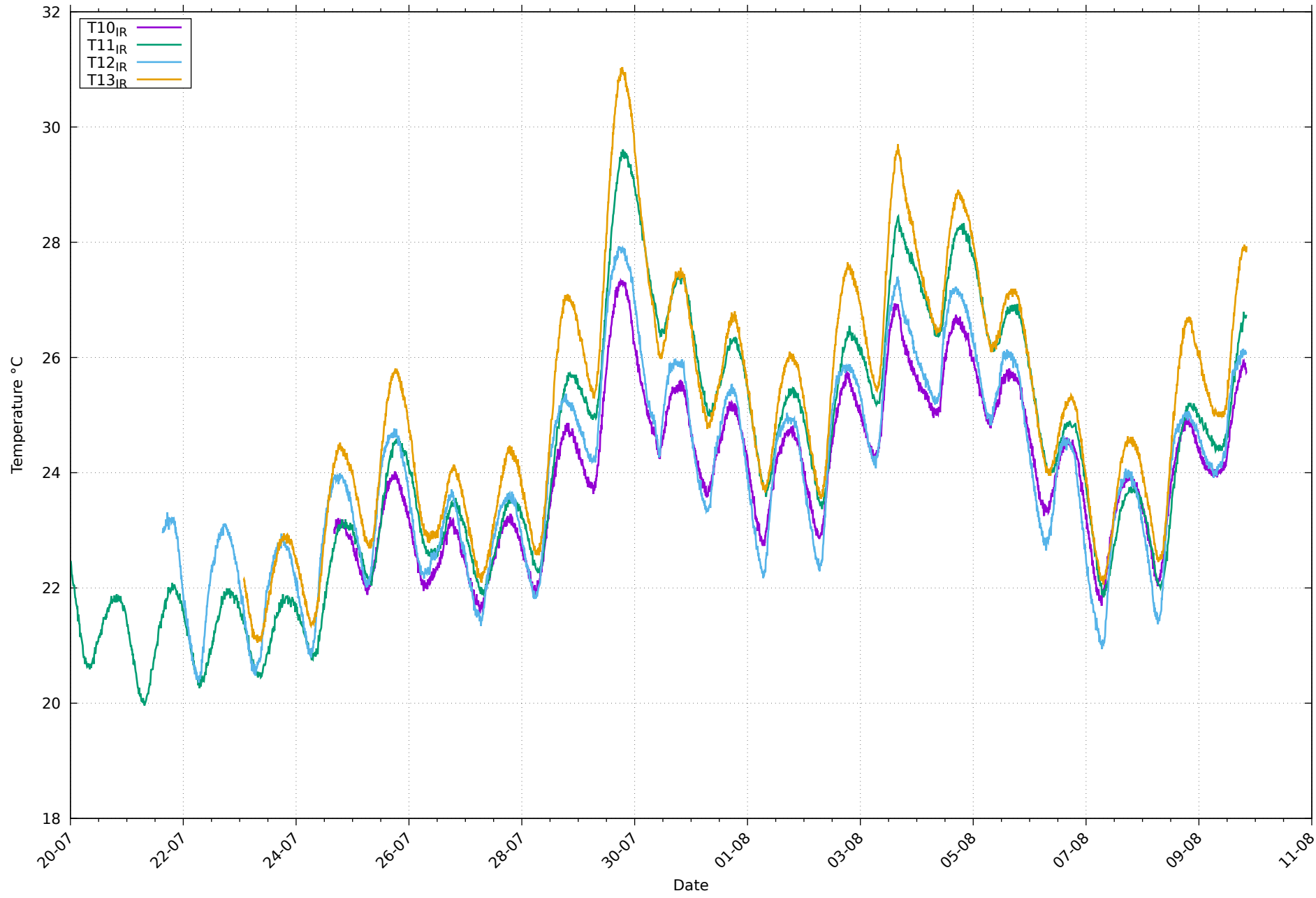
Températures de paroi IR au 09/08/2026
