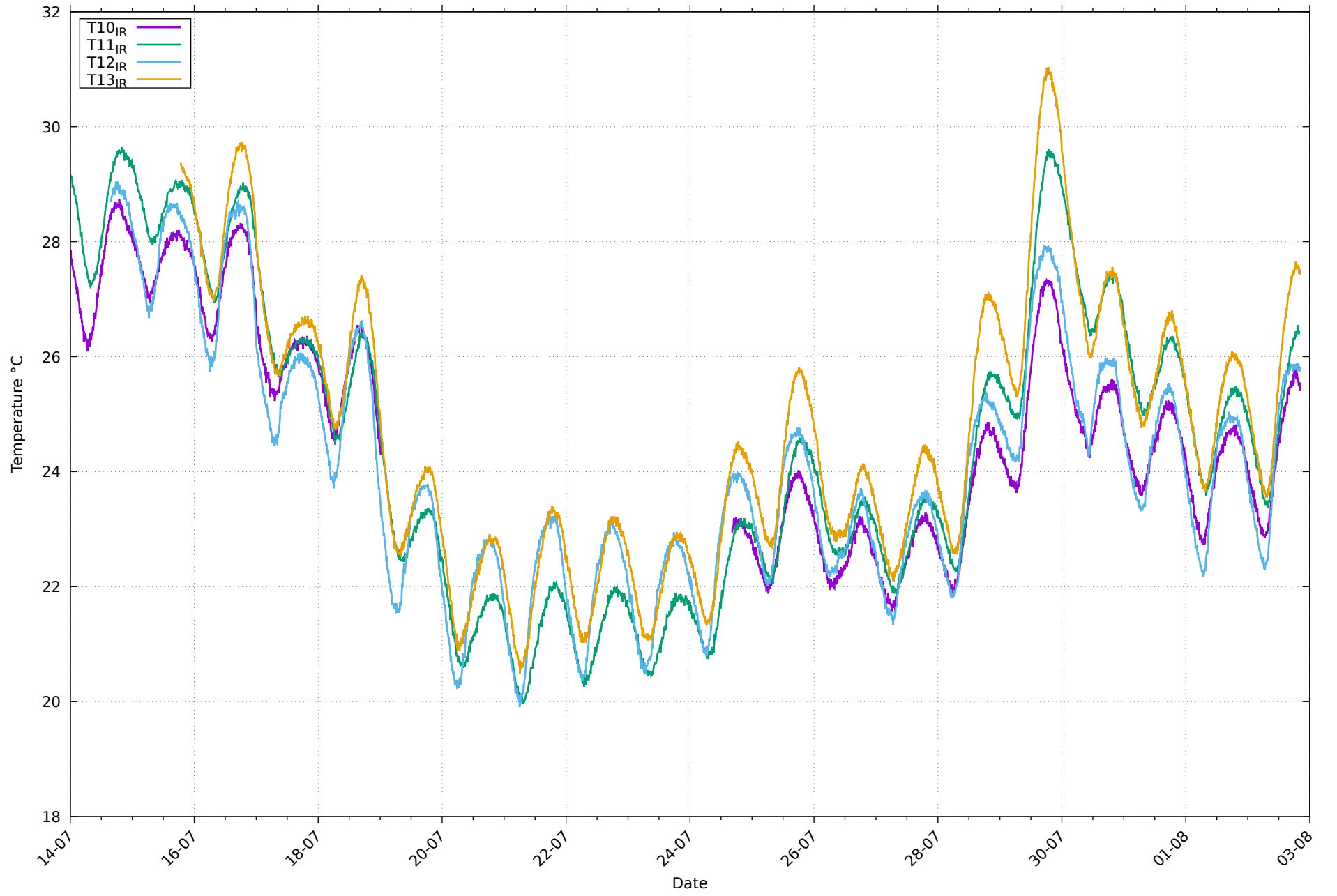
Températures de paroi IR au 02/08/2026
