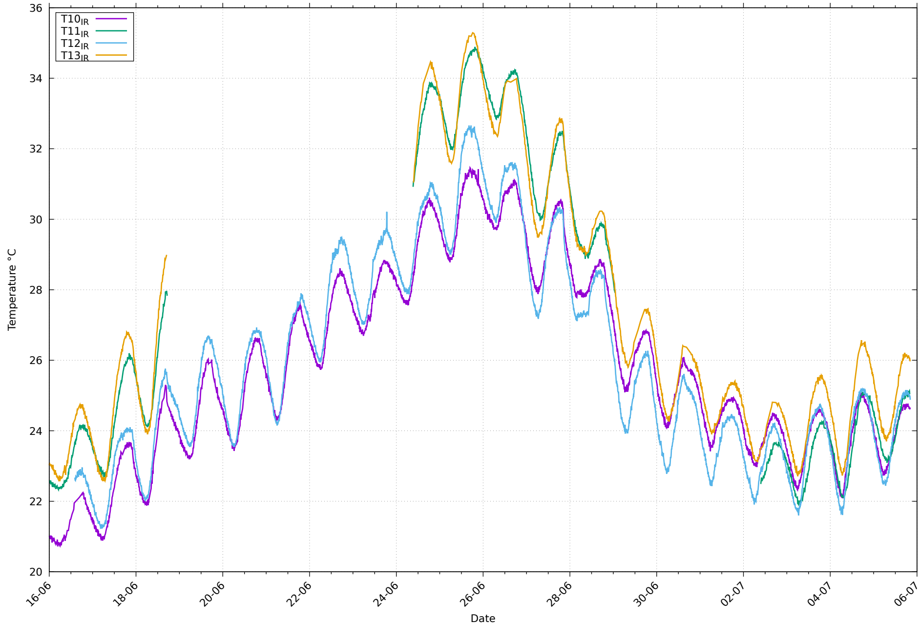
Températures de paroi IR au 05/07/2026
